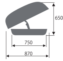
イノーシャドウ18 BRM1800 限定品 製品重量: 20kg
