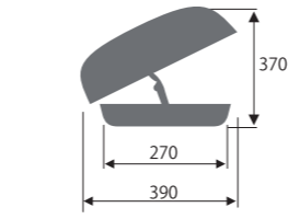
NEW ロッドボックス IF44 製品重量: 12kg
