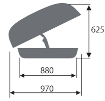
イノールーフボックス BRM466 製品重量: 22.5kg
