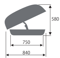
イノールーフボックス33 BRQ33 製品重量: 15kg
