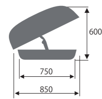
イノーシャドウ16 BRQ124 製品重量: 19kg
