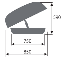
イノーWEDGE PLUS 864 BRM864 製品重量: 21.5kg
