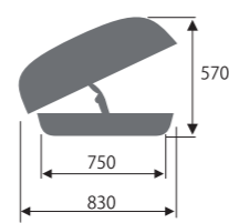
イノールーフボックス55/56 BRQ55 製品重量: 15.5kg
