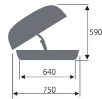
リッジトランク BRW240 製品重量: 9kg
